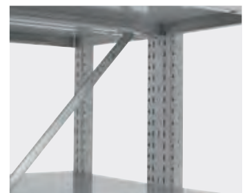
Stabilität durch Feld-Kreuzdiagonale.
