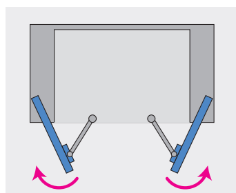
Funktionsprinzip Einschwenktüren.
