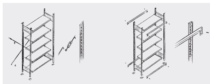
Versteifung des Regals wahlweise mit Feld-Kreuzdiagonale (links) oder mit Breitenriegeln (rechts).
