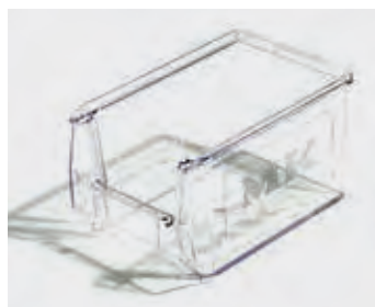
Kastentyp mk 4 transparent. 3,3 Liter Fassungsvermögen. Höhe 130 mm/ Breite 148 mm/Länge 240 mm.
