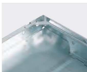
Konstruktiv aufwendige Fachbodenecke mit durchgehender Überlappung durch den zusätzlichen Eckensteg.
