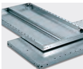
Fachboden mit Fachbodenversteifung (UVR) bei Belastungsgruppe 300 kg.
